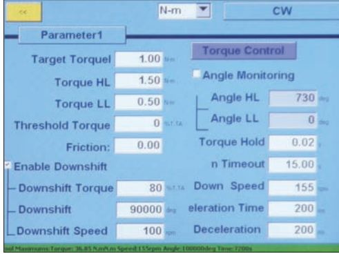
sıkma parametre ayarı arayüzü
