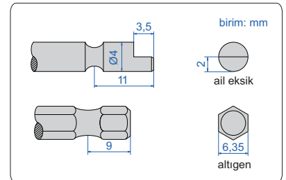
tornavida kafası (opsiyonel) (özellikle: çapraz, düz başlı, altıgen, yıldız şekilli)
